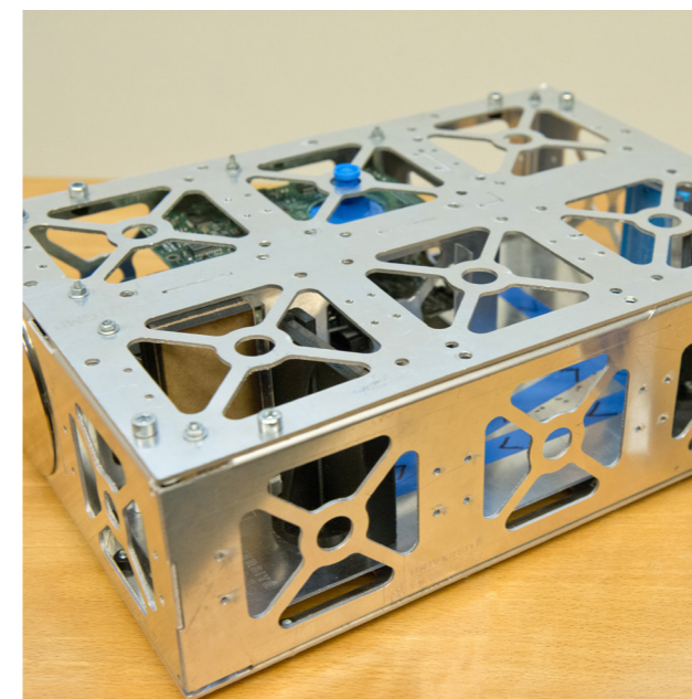
Maquette de l'instrument ATISE
